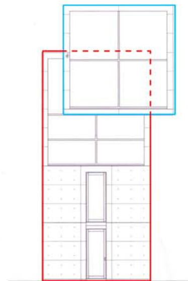
prospetto sud
