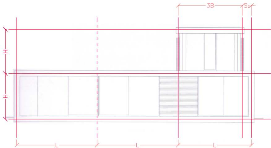
prospetto sud
