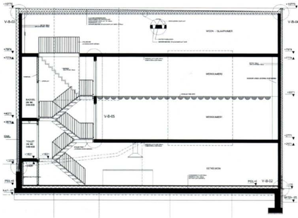
Sección longitudinal BB / Longitudinal section BB
