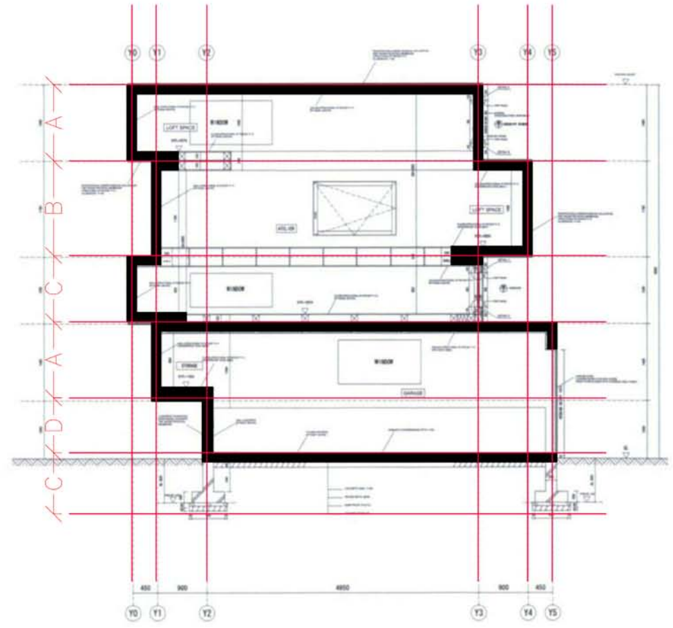
Sección transversal B-B / Cross section B-B
