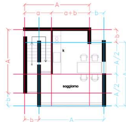
pianta piano terzo
