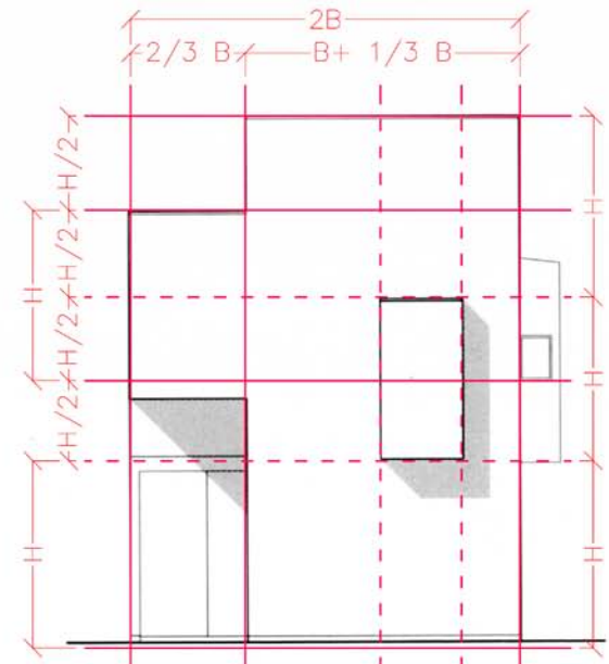
prospetto sud
