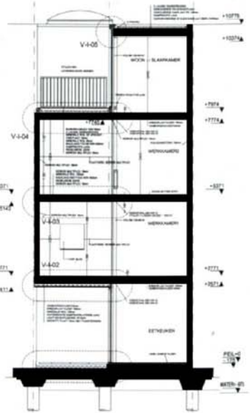
Sección transversal II / Cross section II
