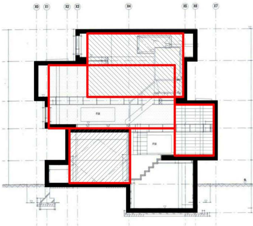
Sección transversal A-A / Cross section A-A
