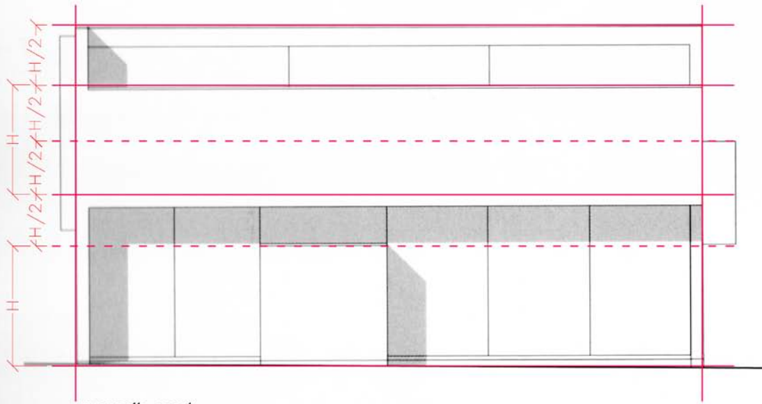
prospetto ovest
