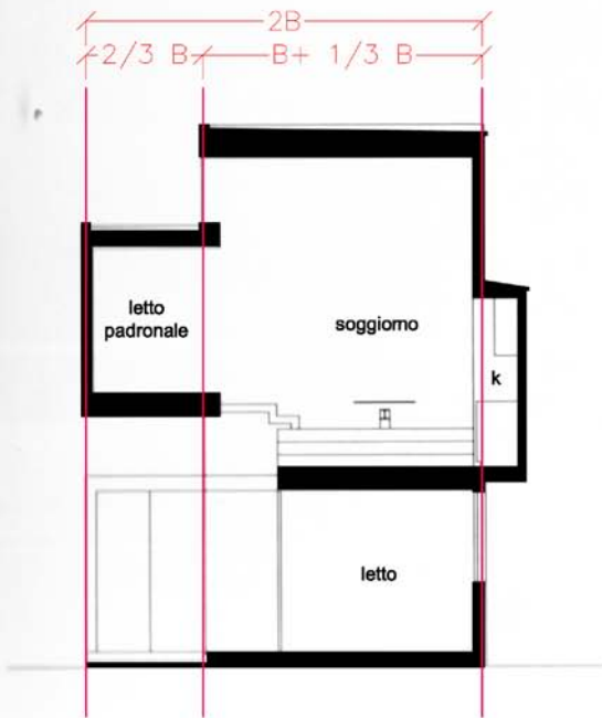
sezione trasversale
