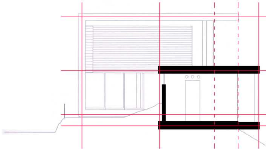
sezione trasversale
