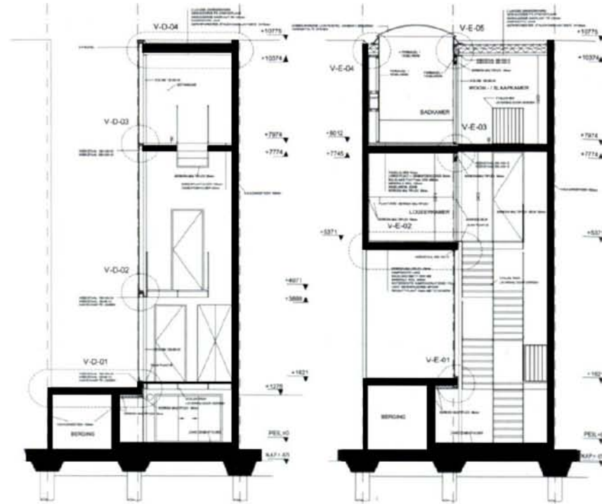
Sección transversal DD / Cross section DD
