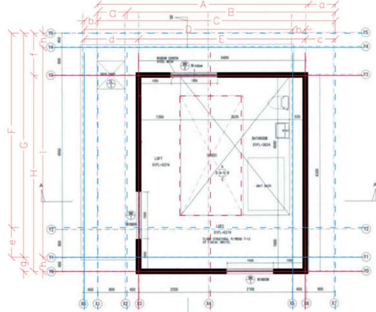
Planta cuarta / Fourth floor plan
