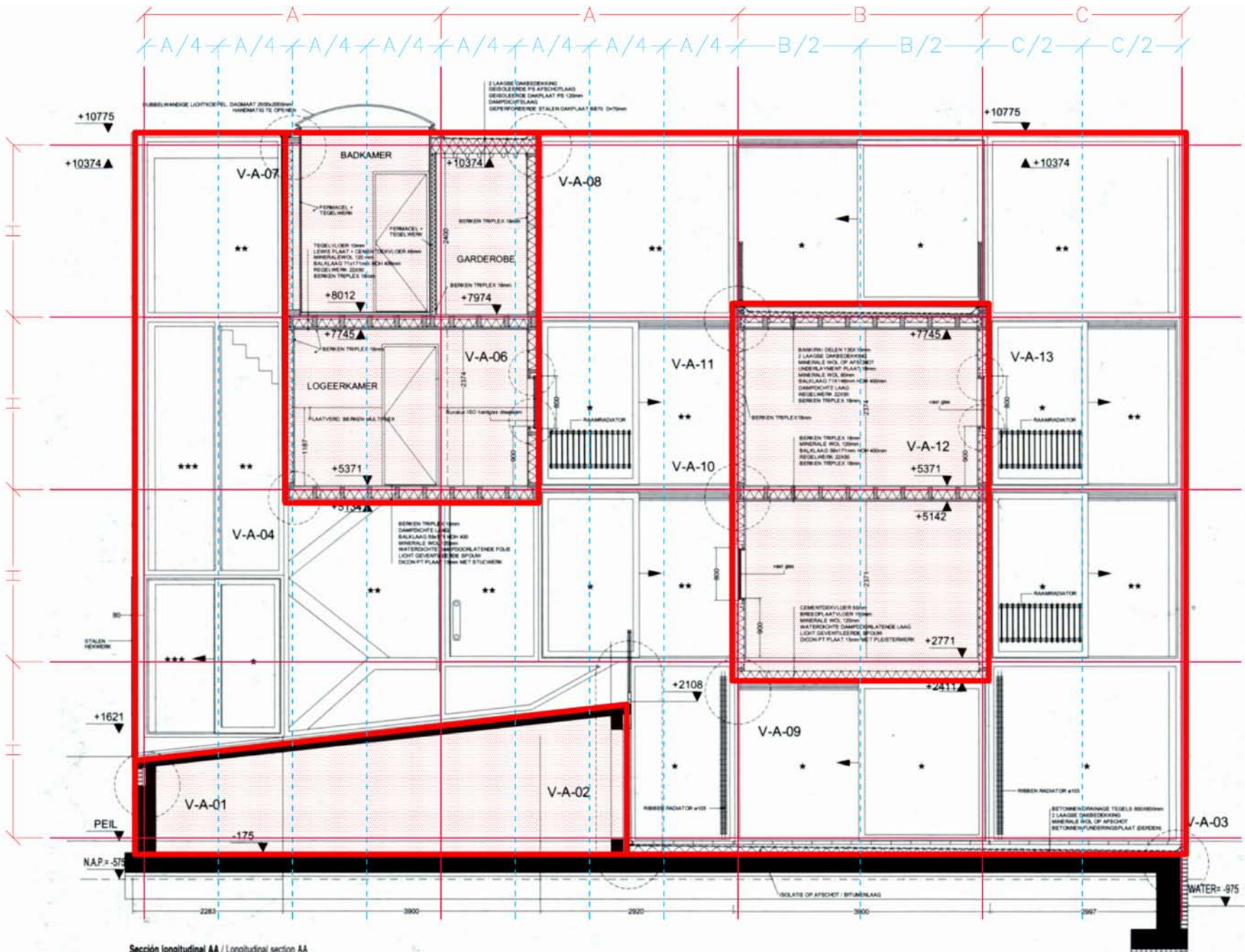
Sección longitudinal AA / Longitudinal section AA
