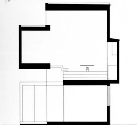
sezione trasversale
