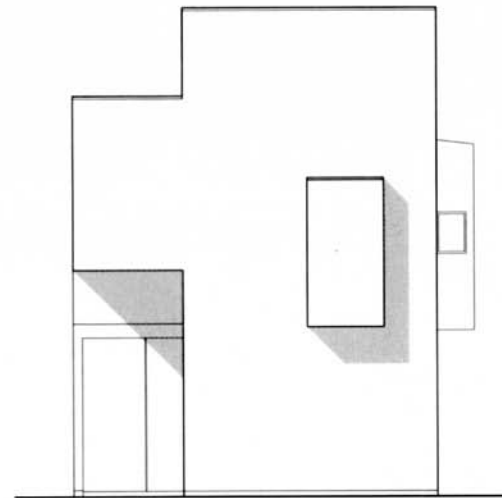
prospetto sud
