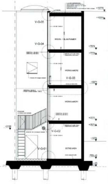
Sección transversal GG / Cross section GG
