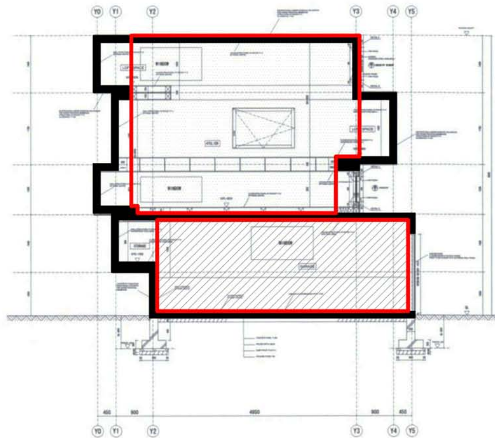
Sección transversal B-B / Cross section B-B
