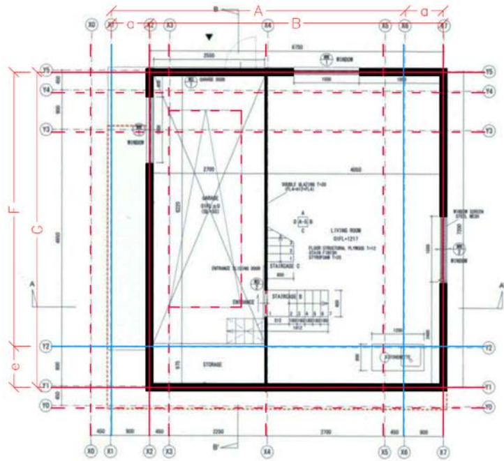
Planta primera / First floor plan
