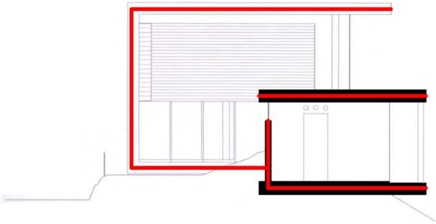
sezione trasversale
