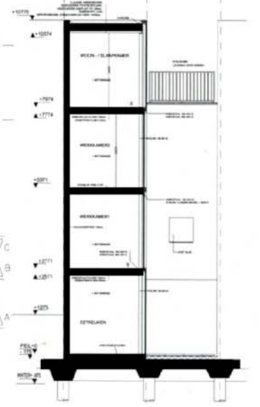
Sección transversal HH / Cross section HH
